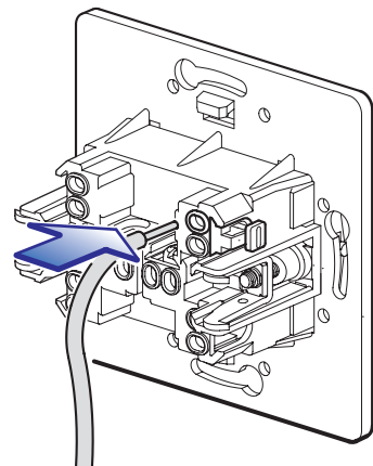
INSTALARE CU ȘURUBURI INSTALLATION WITH SCREWS
