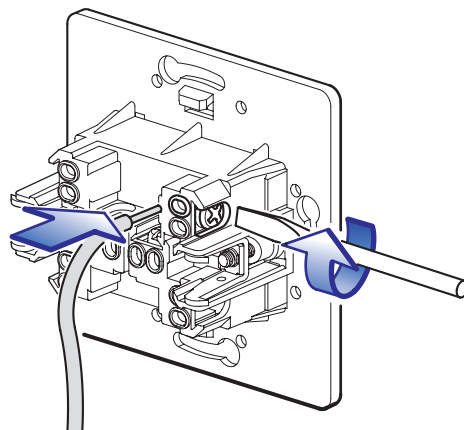
INSTALARE CU ȘURUBURI INSTALLATION WITH SCREWS
