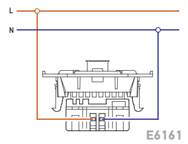
USB töltő csatlakozó aljzat USB charger
