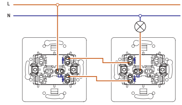
Alternatív (váltó) kapcsoló, két huzalozás (bal és jobb) Alternative switch, two wiring executions (left and right)
