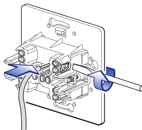
CSAVARRAL TÖRTÉNŐ BESZERELÉS INSTALLATION WITH SCREWS
