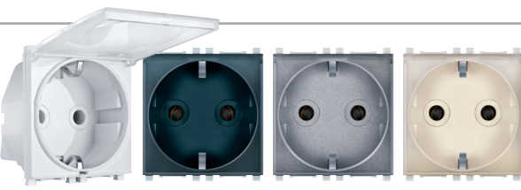
74153.xT Priključnica dvopolna sa transparentnim poklopcem 16A 250V- EXP 2M Double-pole socket outlet with transparent cover 16A 250V- EXP 2M
