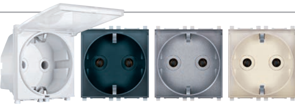
74153.xT Priključnica dvopolna sa transparentnim poklopcem 16A 250V~ EXP 2M 2 pole socket outlet with transparent cover 16A 250V~ EXP 2M
