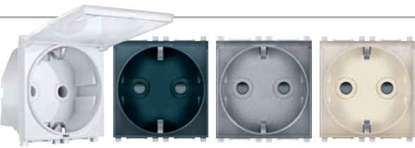
74154.xT Priključnica dvopolna sa transparentnim poklopcem i zaštitom kontakata 16A 250V~ EXP 2M 2 pole socket outlet with transparent cover and safety shutter 16A 250V~ EXP 2M
