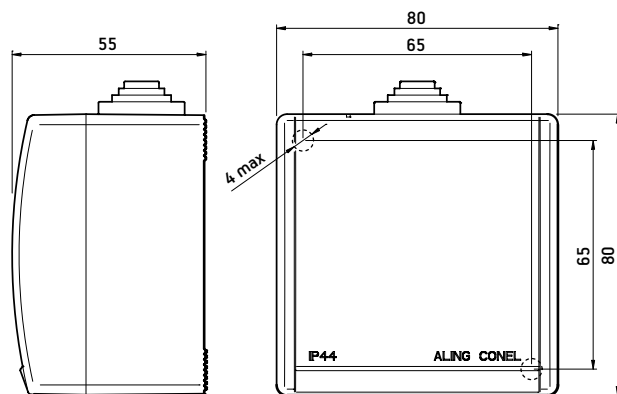
Priključnica tropolna Three-pole socket outlet
