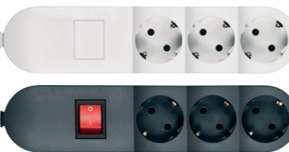
4403.x Priključnica prenosna trostruka, bez kabl, sa dvopolnom indikatorskom sklopkom. max 3600W, 3x16A 250V~
