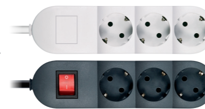
Priključnica prenosna nerastavna trostruka, max 3600W, 3x16A 250V~ Triple portable socket outlet unwireable, max 3600W, 3x16A 250V~
