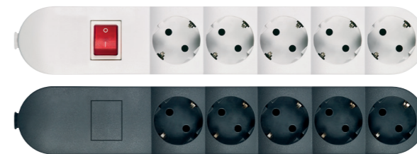
4405.x Priključnica prenosna petostruka, bez kabl, sa dvopolnom indikatorskom sklopkom. max 3600W, 5x16A 250V~
