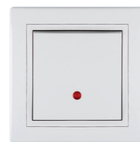
6191.xx Egypólusú kapcsoló, jelzőfényes, 16A 250V~, komplett Single-pole switch with indication 16AX/250V~ • A jelzőfény bekapcsol, ha a kapcsoló be van kapcsolva • Indication is on when the switch is on
